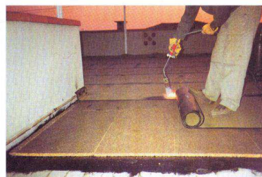
Isolamento di una terrazza
